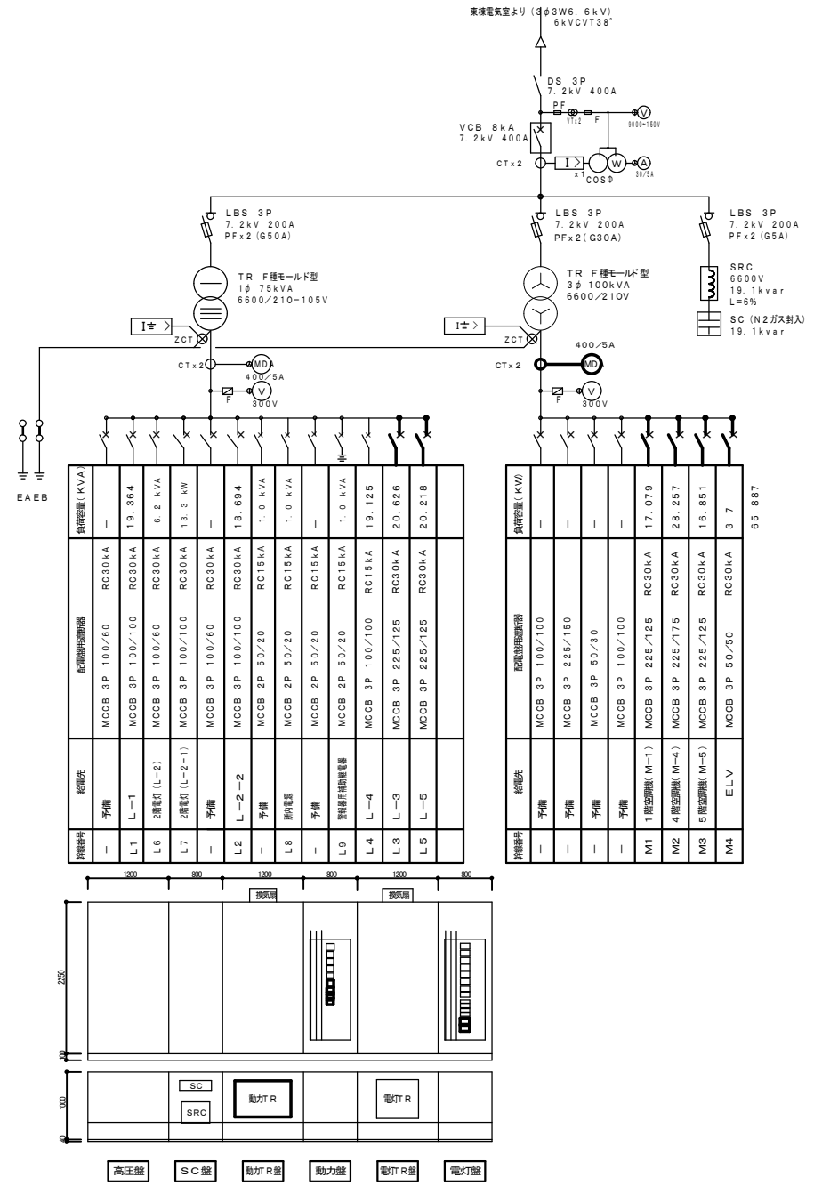
受変電設備 単線系統図
