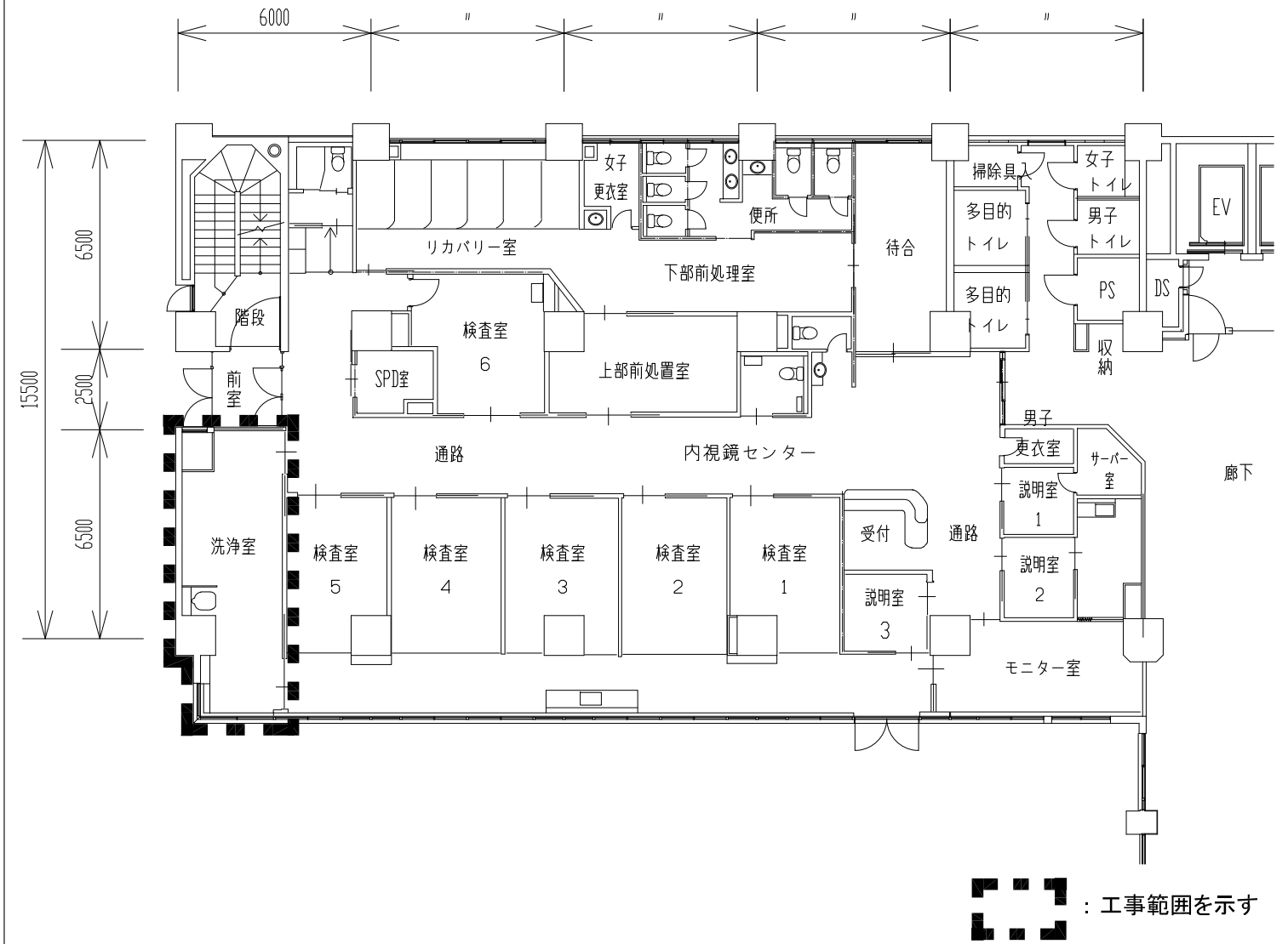
工事範囲平面図（改修後）
