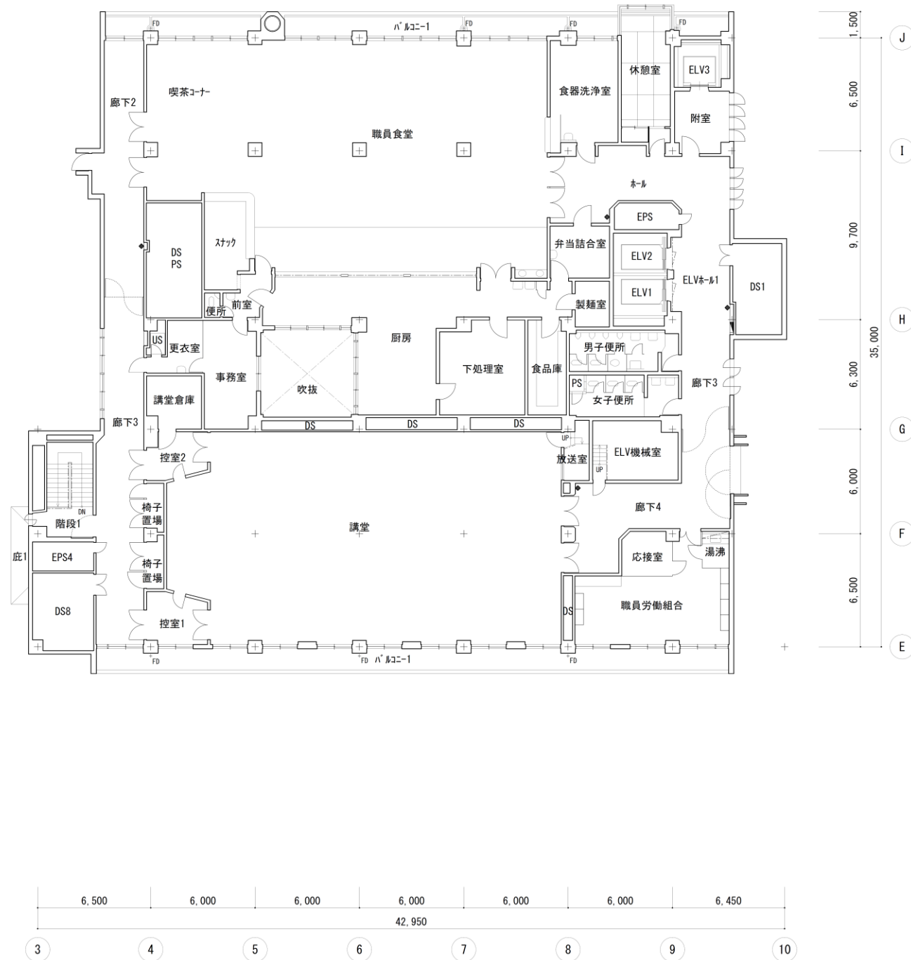
10階平面図
