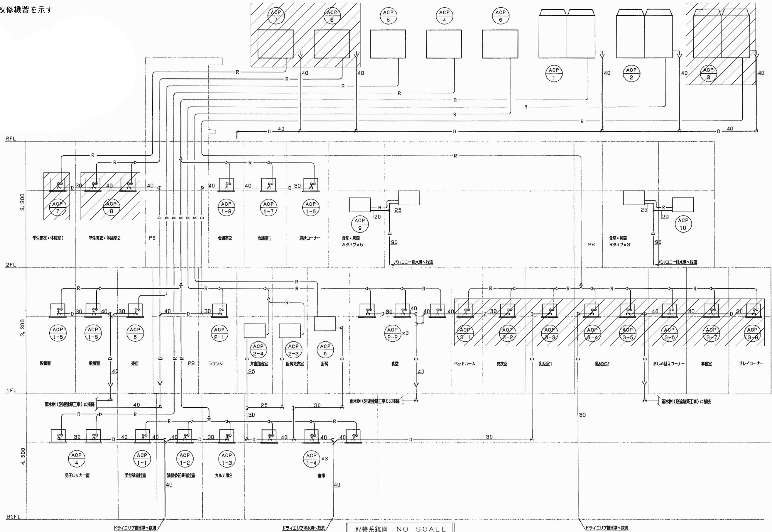
配管系統図 NO SCALE
