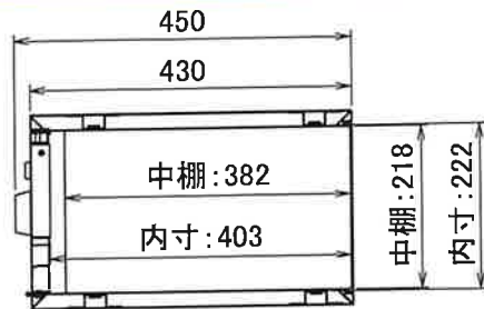
A-A (断面図)
