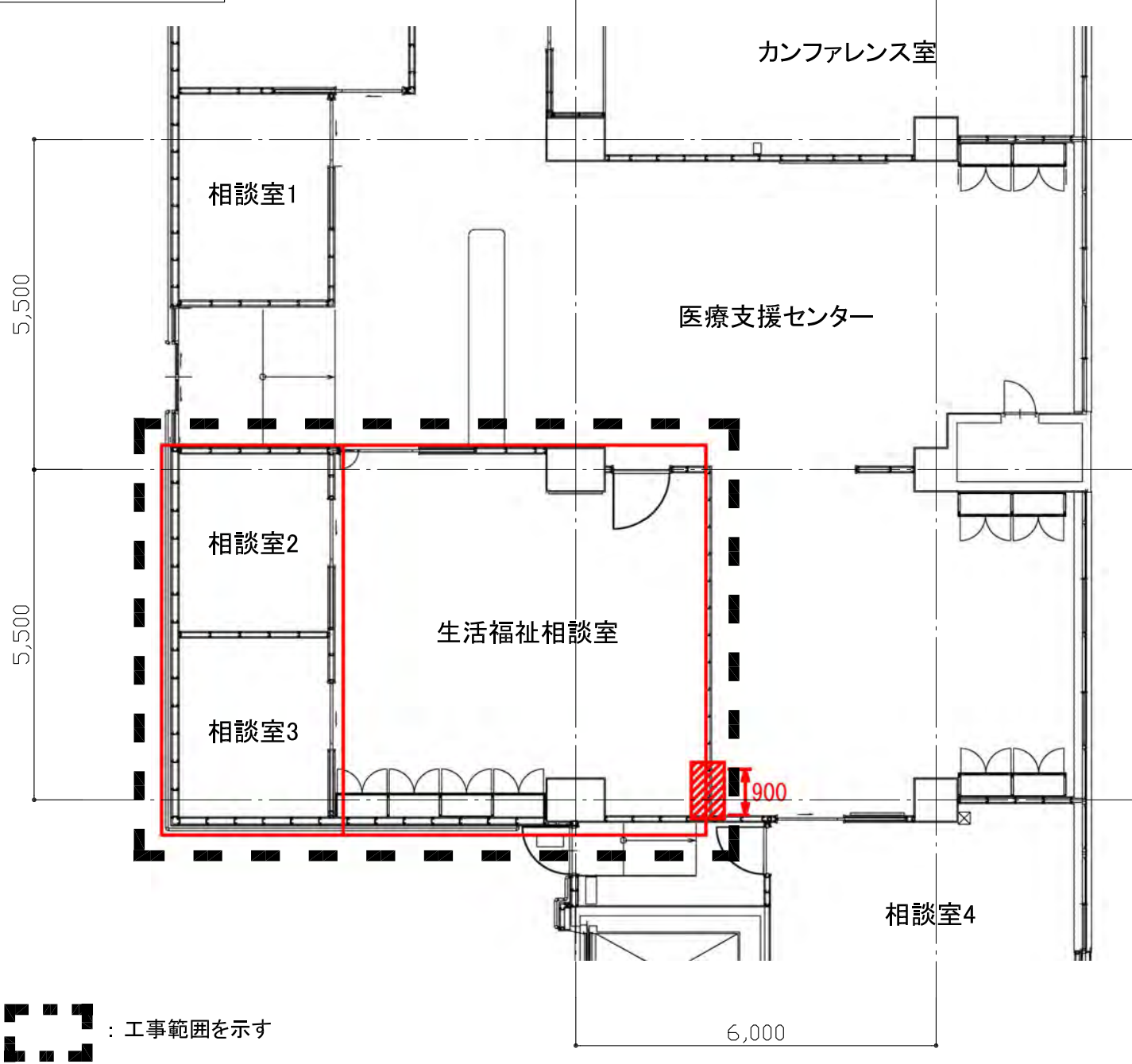
工事範囲平面図（改修前）
