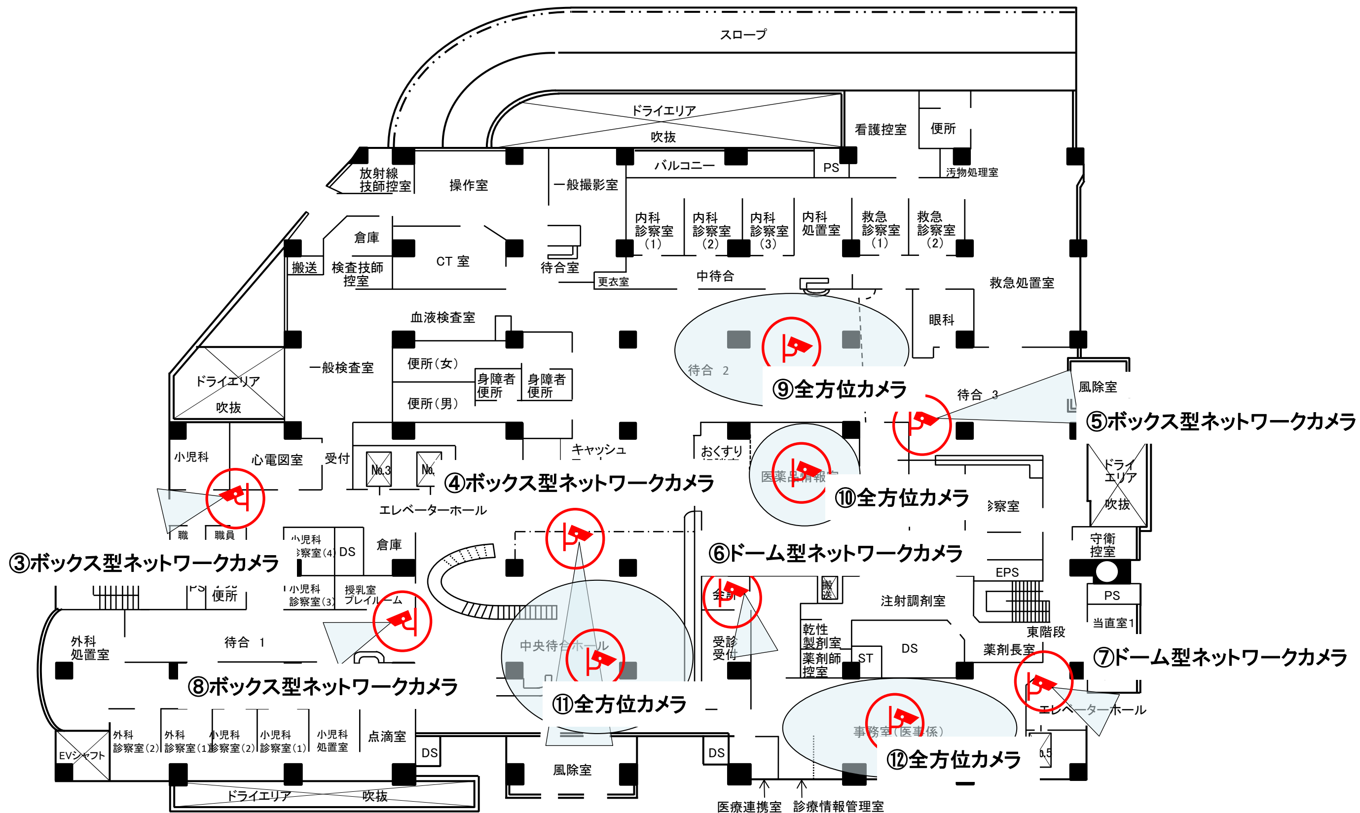
1階平面図
