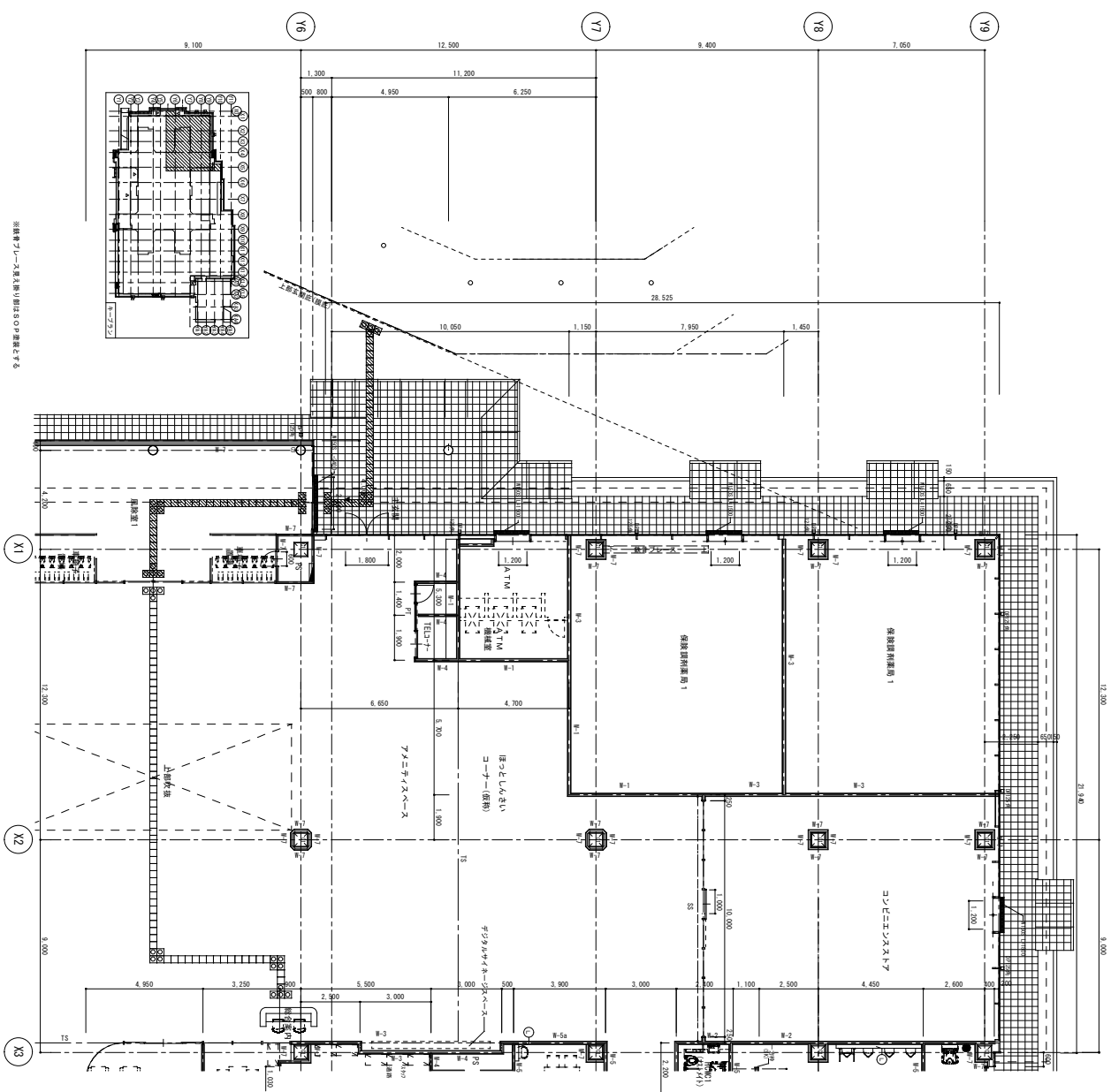
1階平面詳細図① 1/200
