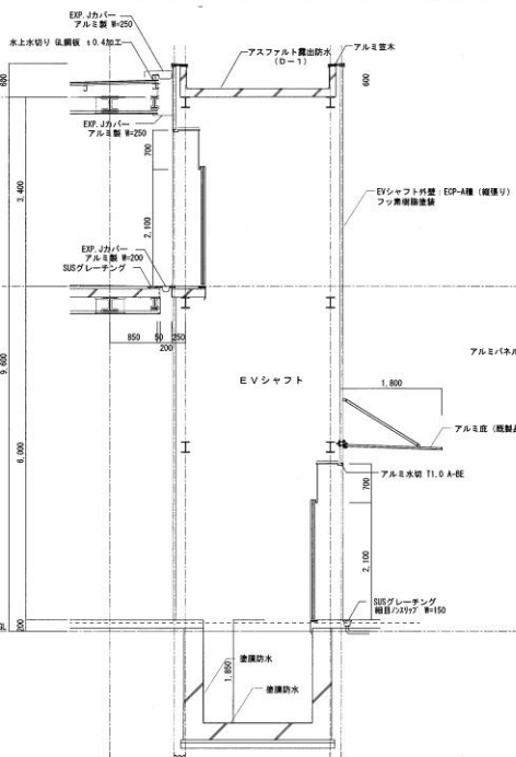
EVシャフト 矩計図 S=1/50
