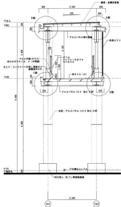
横断橋 矩計図 S=1/50
