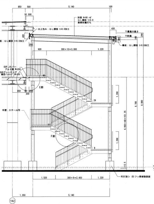
屋外階段 矩計図 S=1/50
