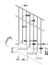
E部詳細図 S=1/20
