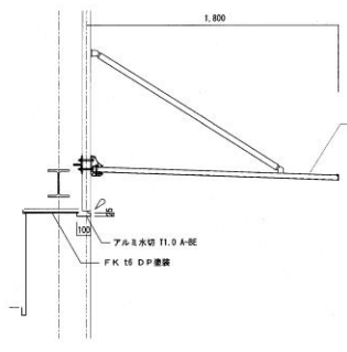
アルミ応詳細図 S=1/20
