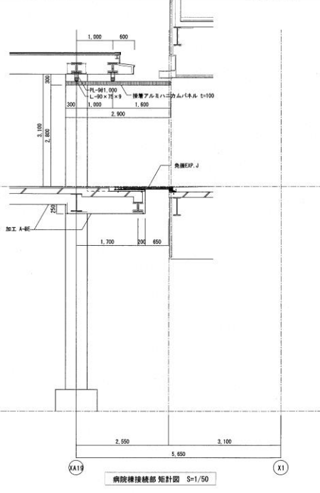
病院棟接続部 矩計図 S=1/50
