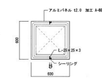
F部詳細図 S=1/20
