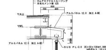
A部詳細図 S=1/20
