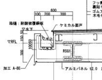
B部詳細図 S=1/20
