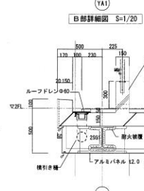
C部詳細図 S=1/20
