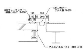
E部詳細図 S=1/20
