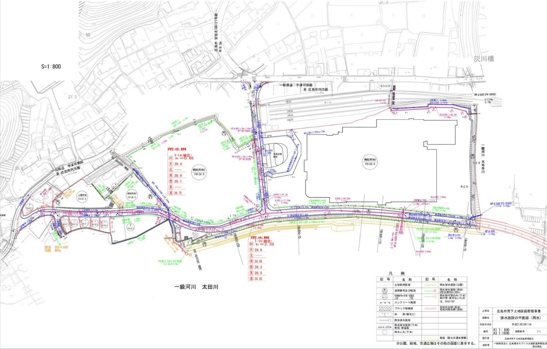
排水施設の平面図（雨水）
