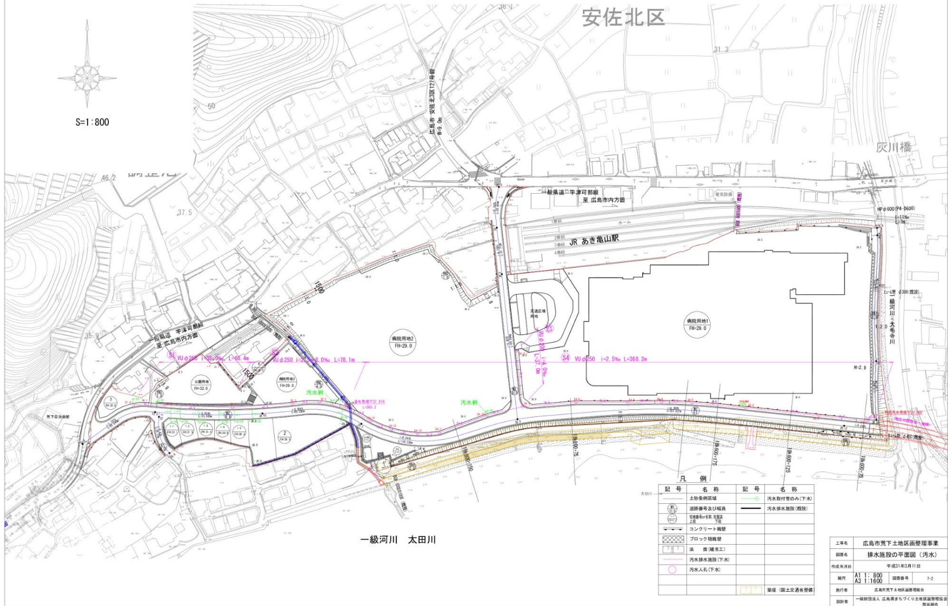
排水施設の平面図（汚水）
