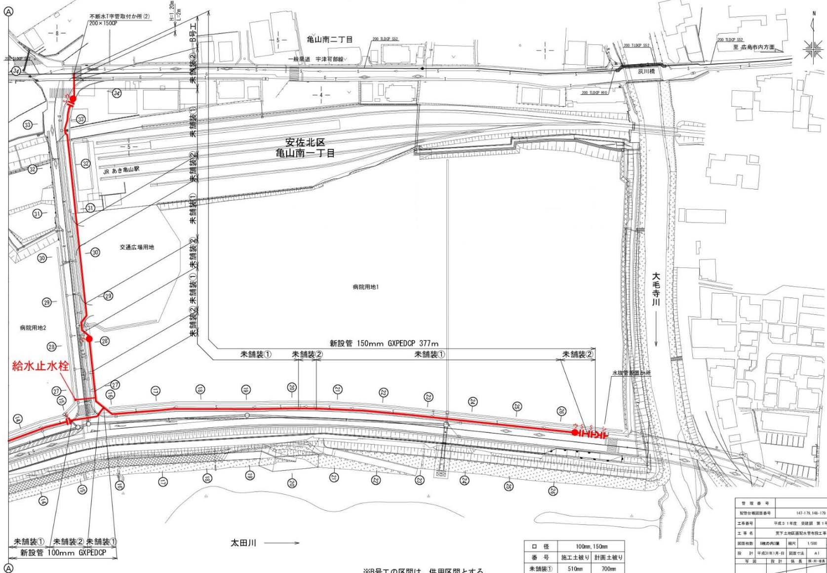
平面圖(2) S=1/500 (水道)
